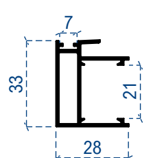
Isıcam kanat profil
