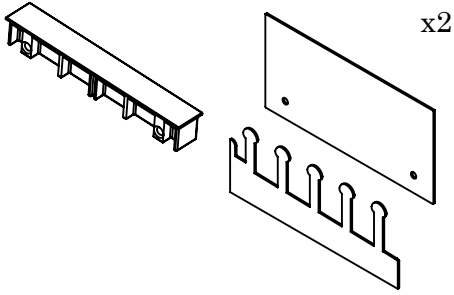
EGE250 5'li Eşikli köşe birleşim
