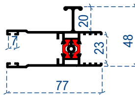
Tek taraflı kol profili
