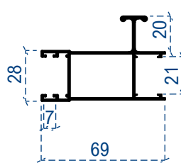
Tek taraflı kol profili
