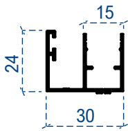
Karşılık profili
