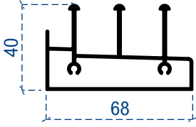
3'lü eşikli alt profil
