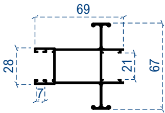
Çift taraflı kol profili
