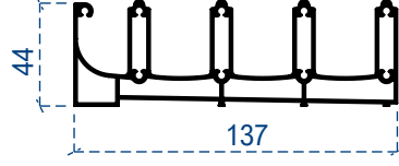
4'lü kasa profili
