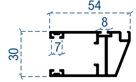
sineklik profili
