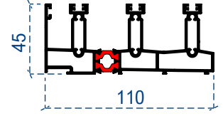
3'lü kasa profili
