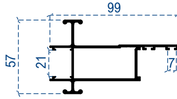
90° Köşe birleşim
