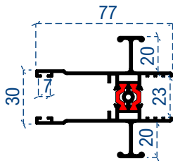
Çift taraflı kol profili
