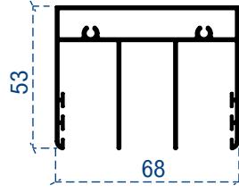
3'lü kasa profili
