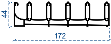
5'li kasa profili
