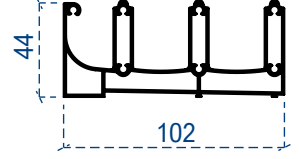
3'lü kasa profili
