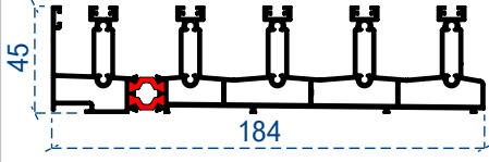
5'li kasa profili
