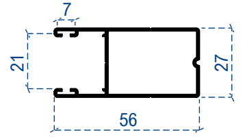
Kilit profili
