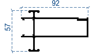
90° Köşe birleşim karşılık
