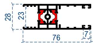
Kanat profil
