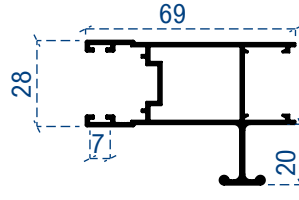
Tek taraflı kol (ispanyolet)
