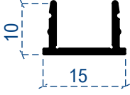
Kapama çitası
