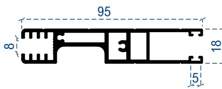
8mm Eşiksiz alt kanat
