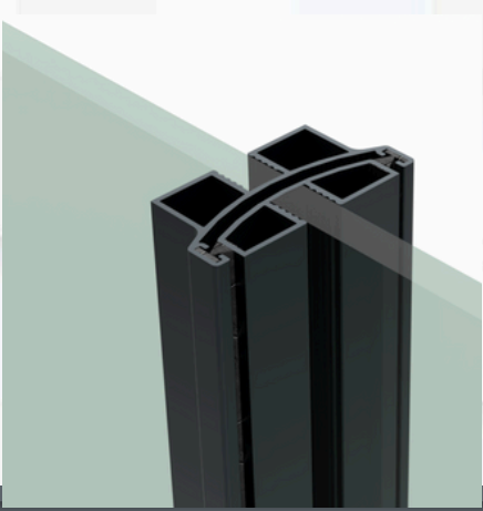
Kasetli ara birleşim seçeneği Cassette interconnection option
