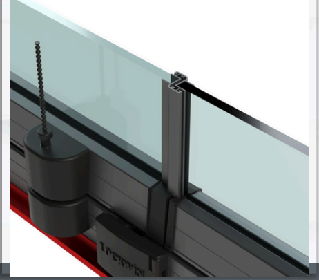
Açılır panel detay Pop-up panel detail
