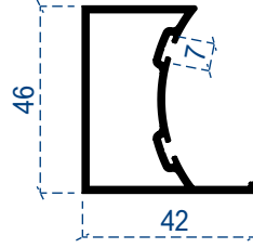
Yan dikme
