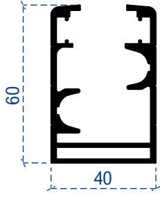
Kasa profili
