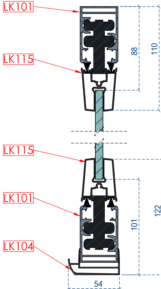
KESİT J-J ÖLÇEK 1 : 2.5
