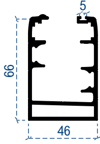
Kasa profili
