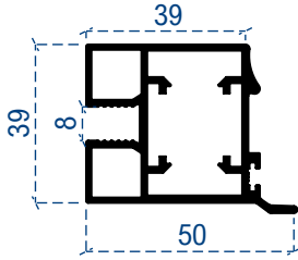
Kol profil
