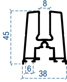
Kanat profil
