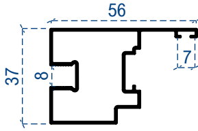
İspanyollet Kol profil
