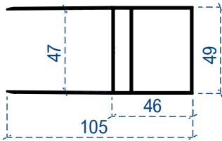
11'lik perdelik
