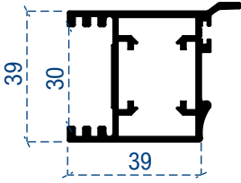
Kol profil
