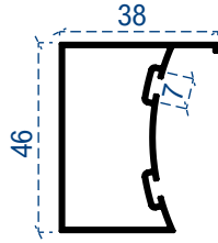
Kanat profil
