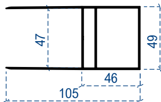
11'lik perdelik
