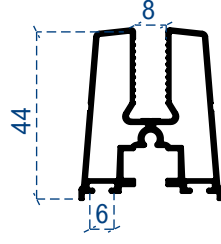
Kanat profil
