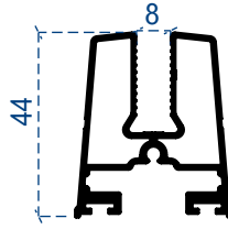
Kanat profil
