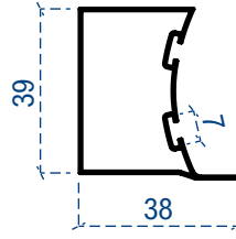
Kasetli Yan dikme
