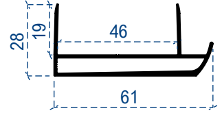
Alt damlalık
