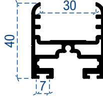
Kanat profil
