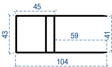
11'lik perdelik
