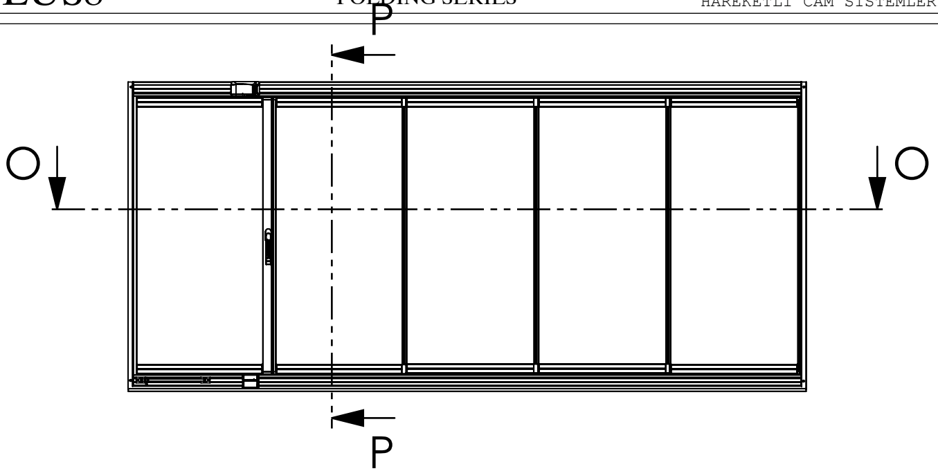
KESİT O-O ÖLÇEK 1 : 2
