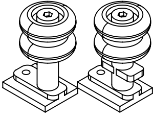
PKS201 Teker
