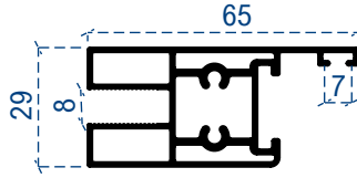
8mm Vasistan yan kanat
