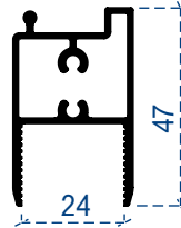
Isıcam Üst kanat
