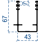
Yan kasa iç U
