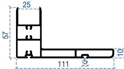
Isıcam yukarı taşıma profili
