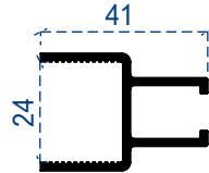
Isıcam Üst kanat
