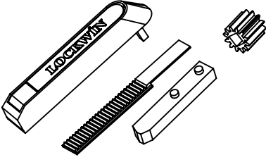
YGS259 Kol mekanizma set
