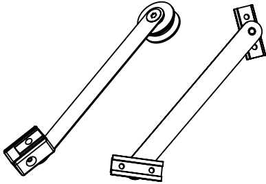
YGS253 Yan kasa kapak
