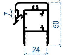
Isıcam kol profili
