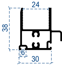
Isıcam alt kanat
