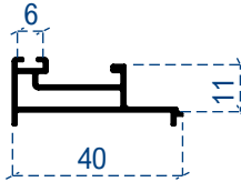
Vasistan adaptör
