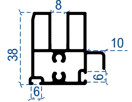
8mm alt kanat
