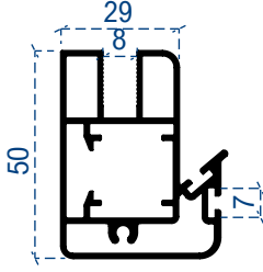
8mm Vasistas kol profil
