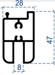
8mm Üst kanat profil
