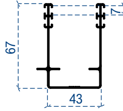
Yan kasa iç U
