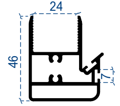
Isıcam kenet profili
