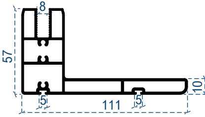
8mm taşıma profili
