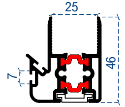
Kenet profili
