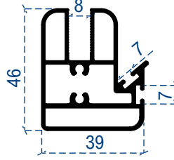
8mm kenet profil
