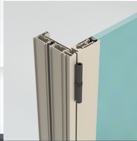
Açılır Kapı detay Sliding Door detail
