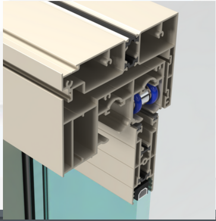
Üst kasa detay Upper case detail
