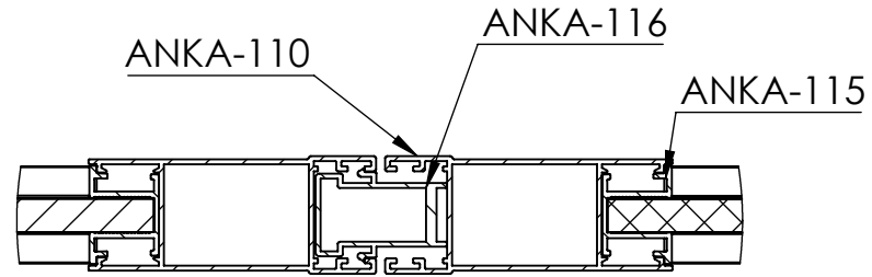
DETAY D ÖLÇEK 1 : 2
