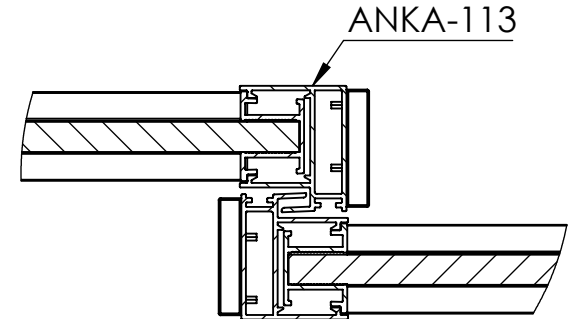
DETAY E ÖLÇEK 1 : 2
