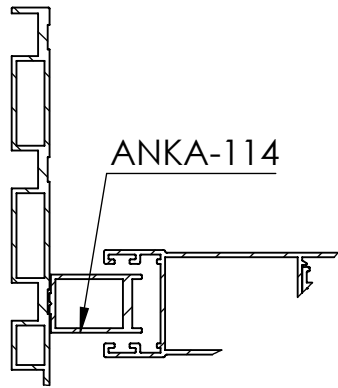
DETAY C ÖLÇEK 1 : 2
